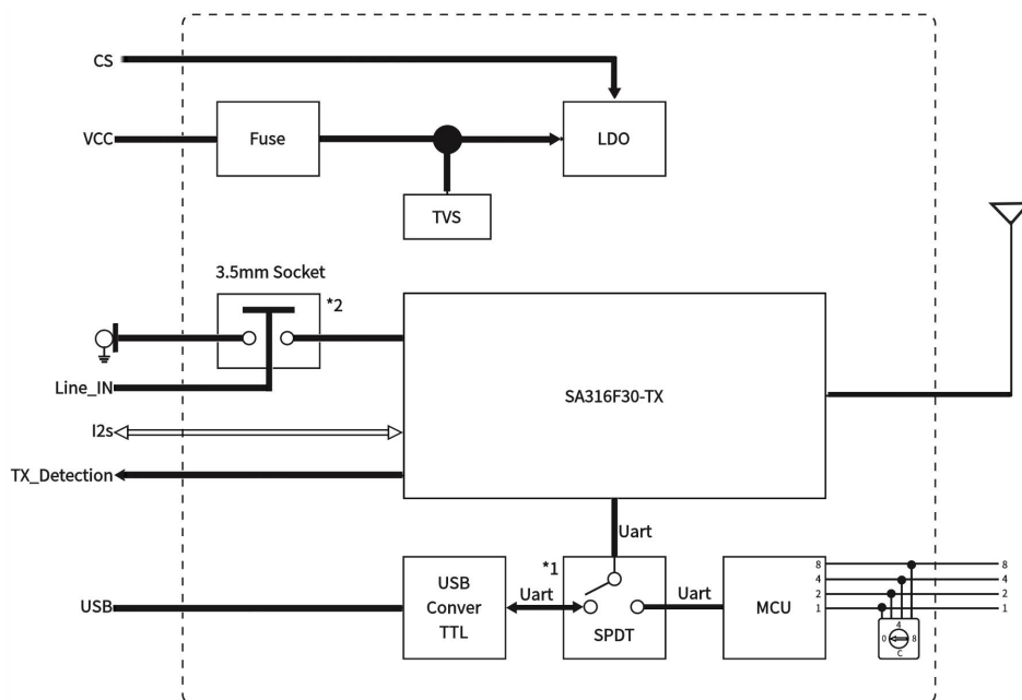
SA326F30-TX 方框图
