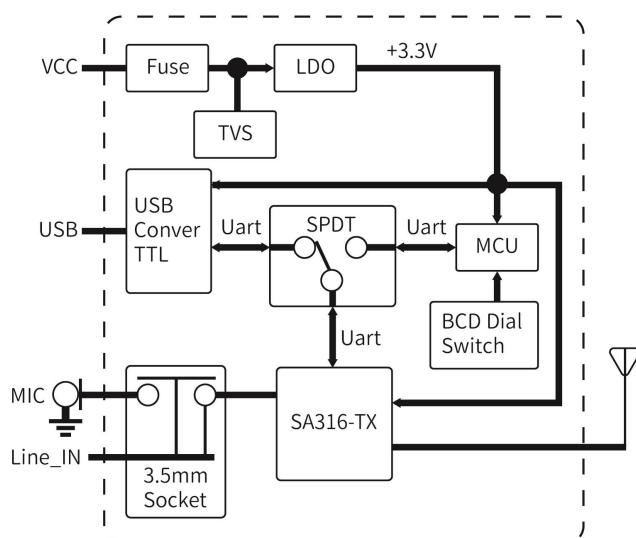
SA326-TX 方框图
